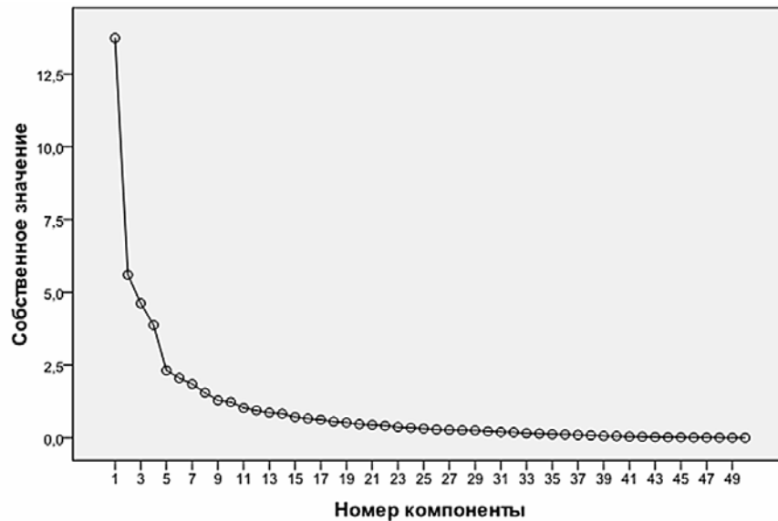
Рисунок 1 — График собственных значений для показателей личностных качеств оперативных сотрудников органов
