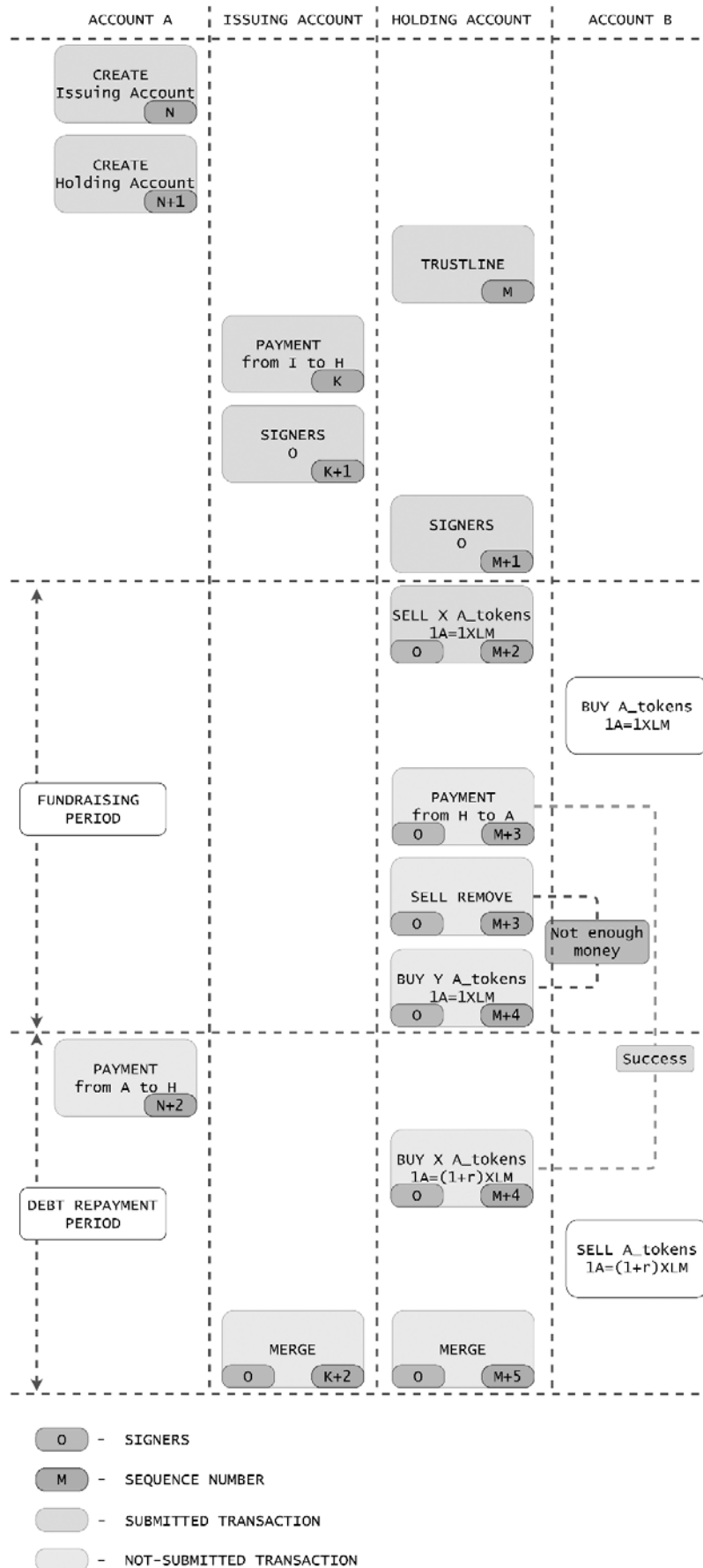
Рисунок 1 — Смарт-контракт кэш-пулинга
